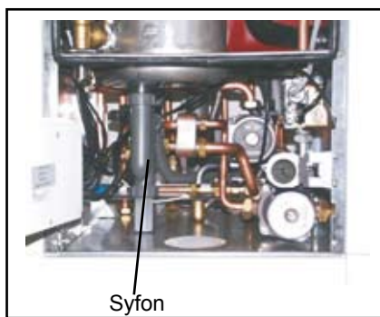
Syfon CGS
