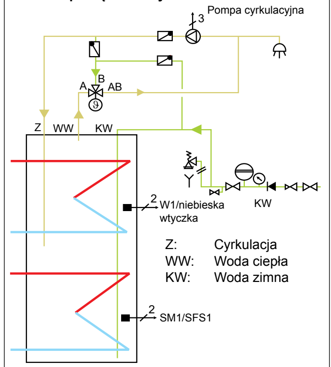
Schemat podłączeniowy:
